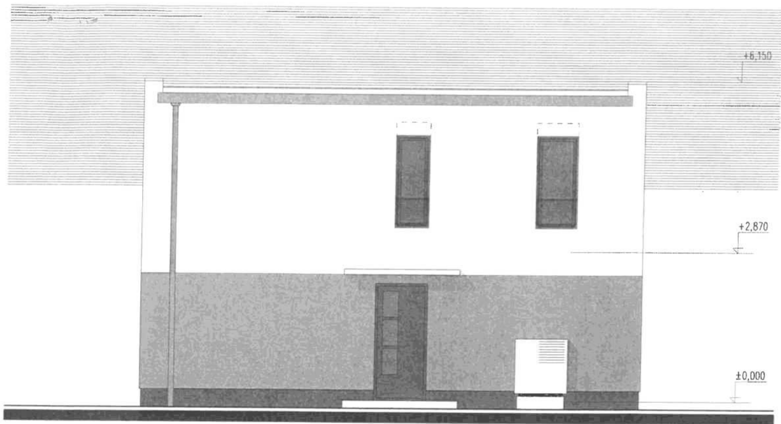
POHLED SEVEROVÝCHODNÍ
