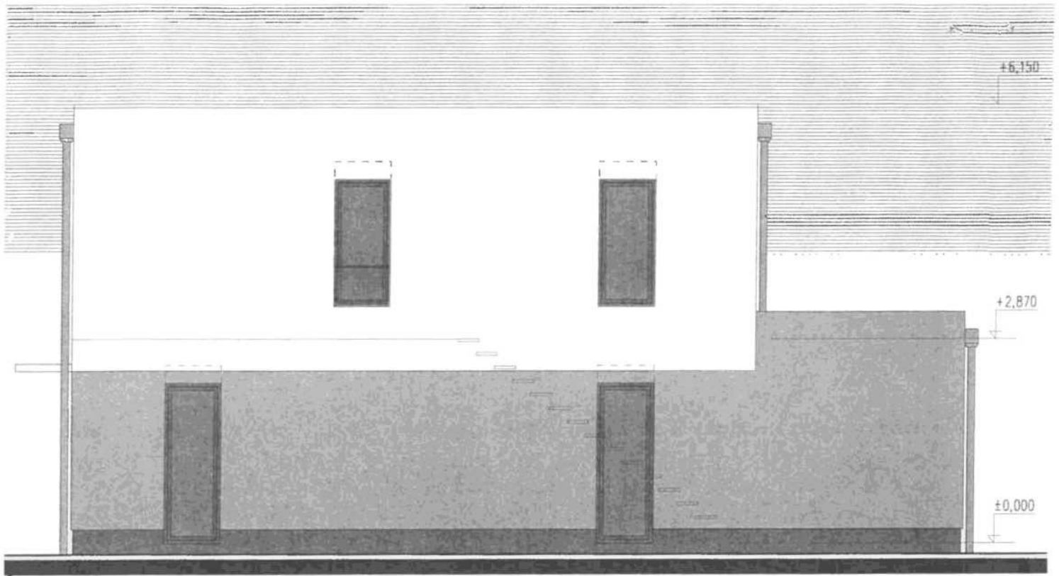
POHLED SEVEROZÁPADNÍ
