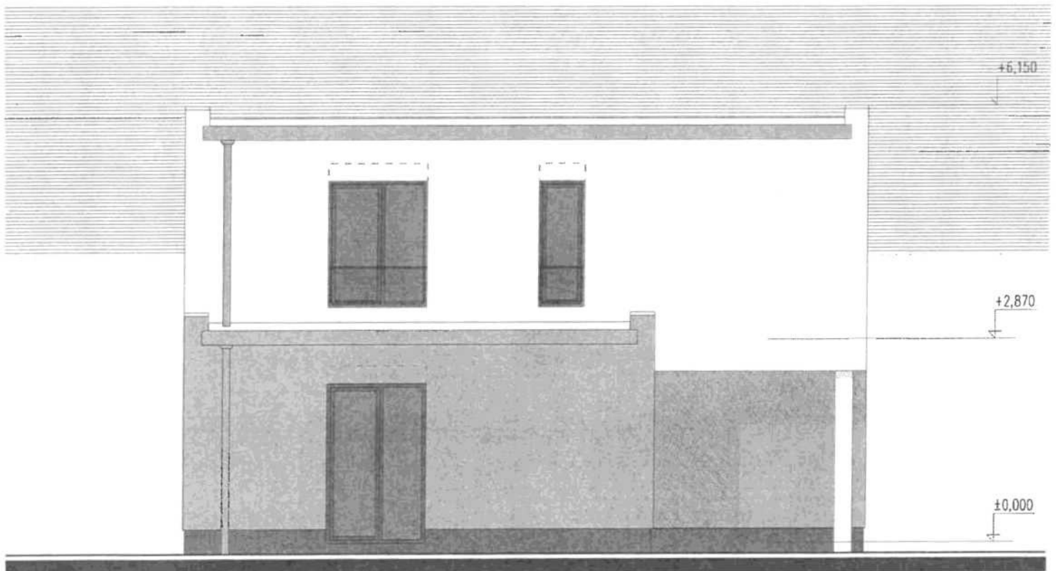
POHLED JIHOZÁPADNÍ
