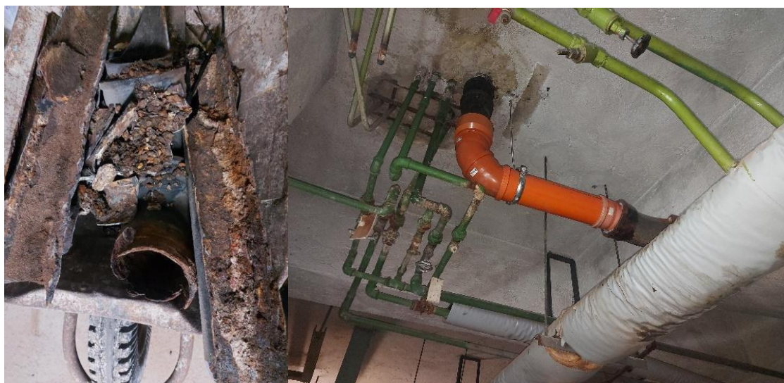
Fotografie č. 13 Prasklé odpadní potrubí sprchy (sportovní hala), VIP místnost, hotel pokoje 5, 6
