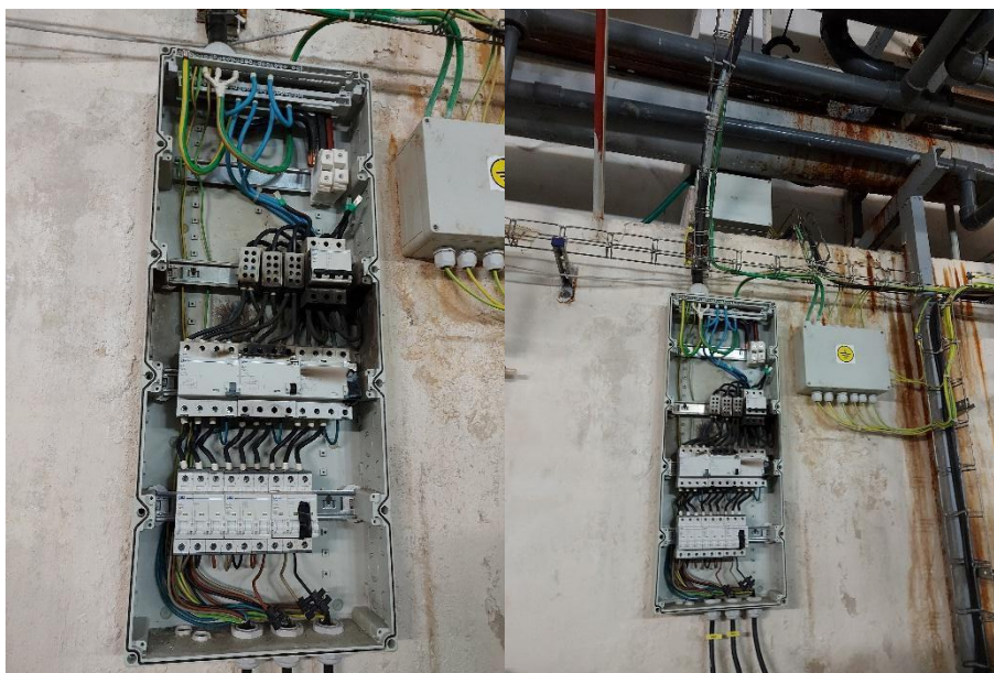
Fotografie č. 12 Prasklé potrubí vířivky a následné zahoření rozvaděče
